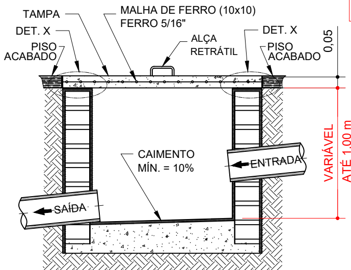
CORTE A-A
